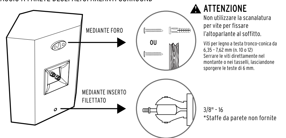
FIGURA 4 FISSAGGIO A PARETE DEGLI ALTOPARLANTI SURROUND
