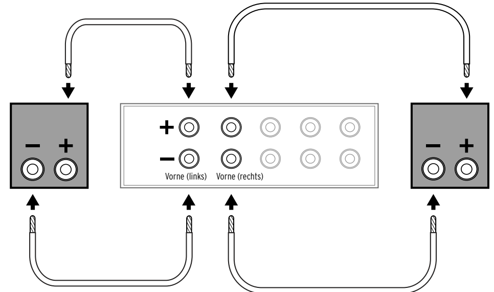
ABBILDUNG 3 STANDARDANSCHLÜSSE
