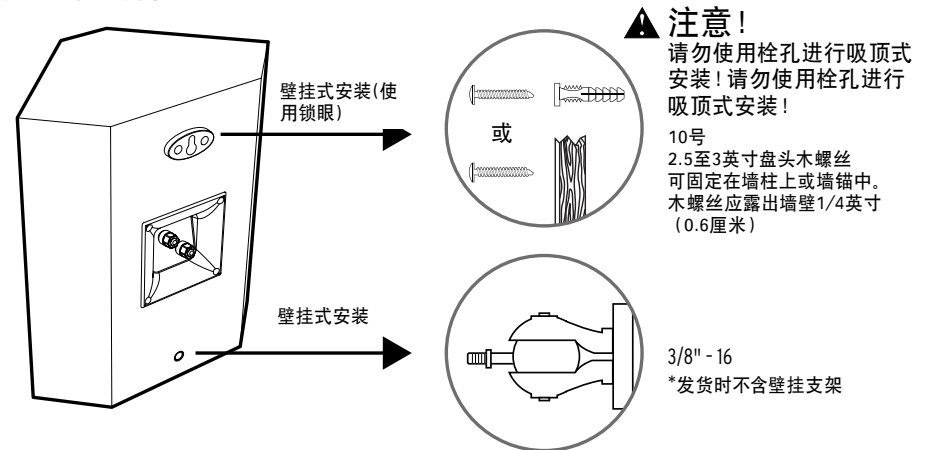
图4 墙面安装环绕音箱
