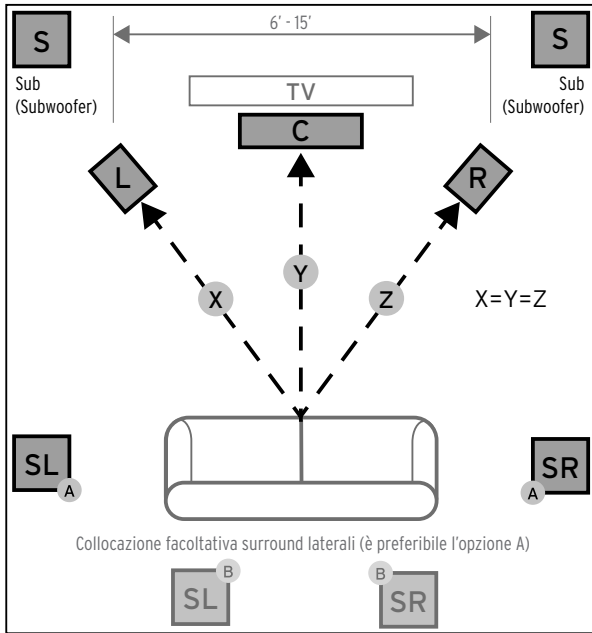
FIGURA 2 CANALE CENTRALE
