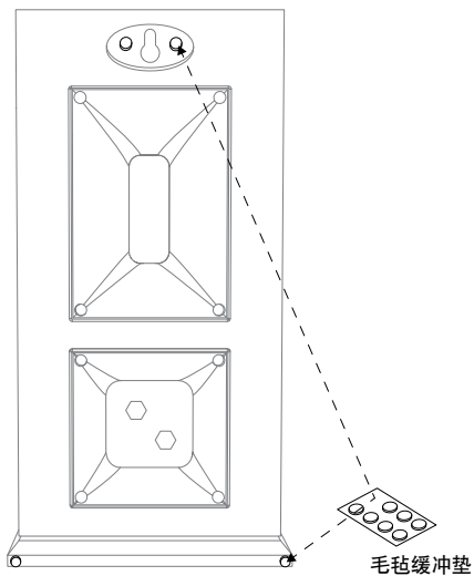
图1 RP-150M 壁挂式安装
