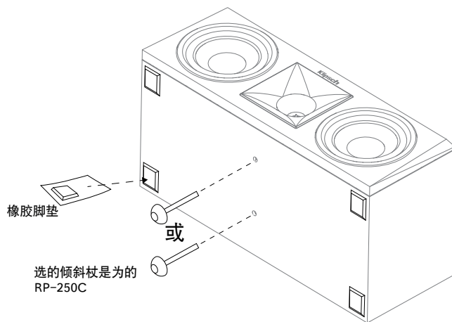
图2 中间声道
