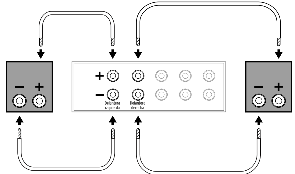
FIGURA 3 CONEXIONES ESTÁNDAR
