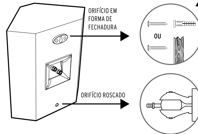
FIGURA 4 INSTALAÇÃO DAS CAIXAS ACÚSTICAS SURROUND EM PAREDE
