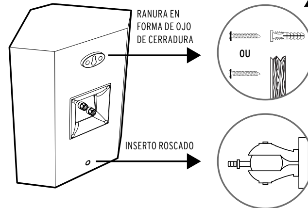
FIGURA 4 MONTAJE DE LOS ALTAVOCES SURROUND EN LA PARED
