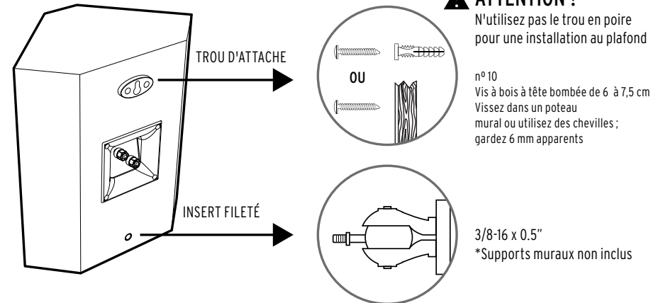
FIGURE 4 MONTAGE MURAL DES ENCEINTES SURROUND
