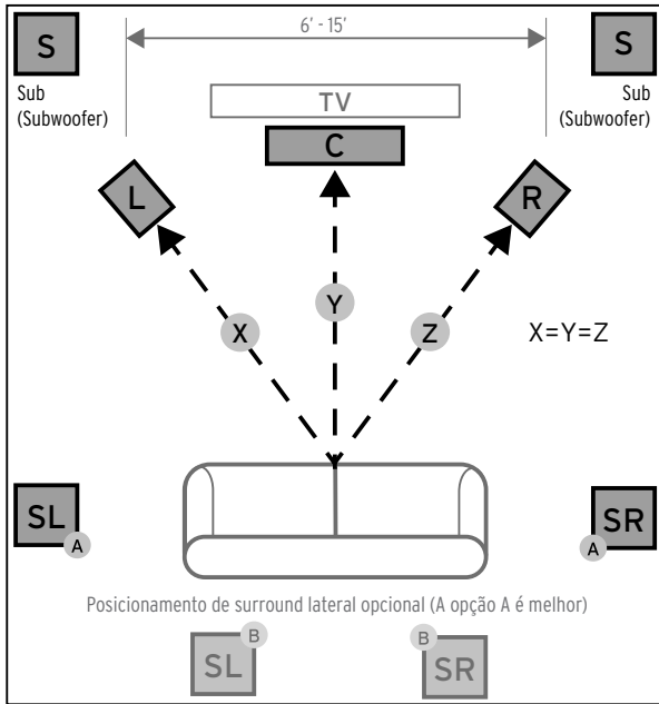
FIGURA 2 CANAL CENTRAL
